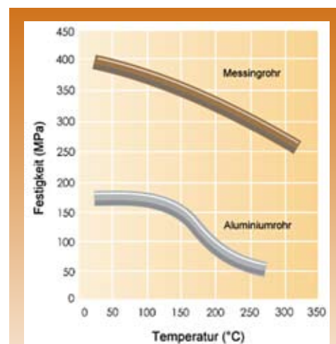
Bild 2: Temperatur abhängige Festigkeit CuZn vs Al
