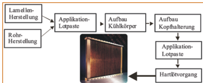
Bild 1: Cupro-Brazo® Verfahren
