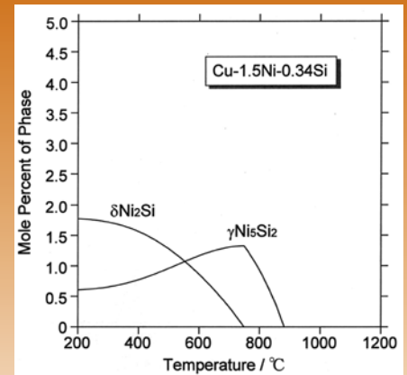
Bild 9: Ausscheidungsphasen [12] für die Legierungszusammensetzung Cu1,5Ni0,34Si (entspricht Legierung 40)
