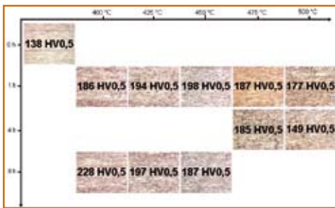
Bild 2: Ergebnisse von verschiedenen Ausscheidungsglühbehandlungen auf die Gefüge und die Härtewerte von ind. lösungsgeglühten und gewalzten Proben der Legierung 40
