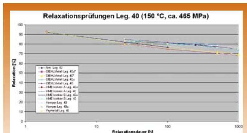
Bild 3: Ergebnisse von Spannungsrelaxationsprüfungen und -versuchen an Proben der Legierung 40.
