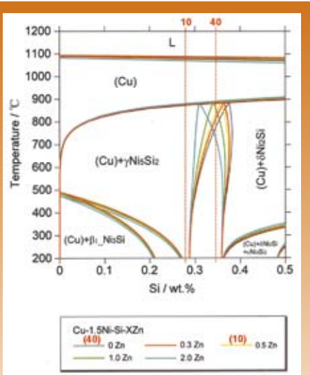
Bild 10: Auswirkung leicht variierender Si-Gehalte und verschiedener Zn-Gehalte auf den quasibinären Ausschnitt Cu-Si bei 1,5Ni im ternären Phasendiagramm Cu-Ni-Si [12]
